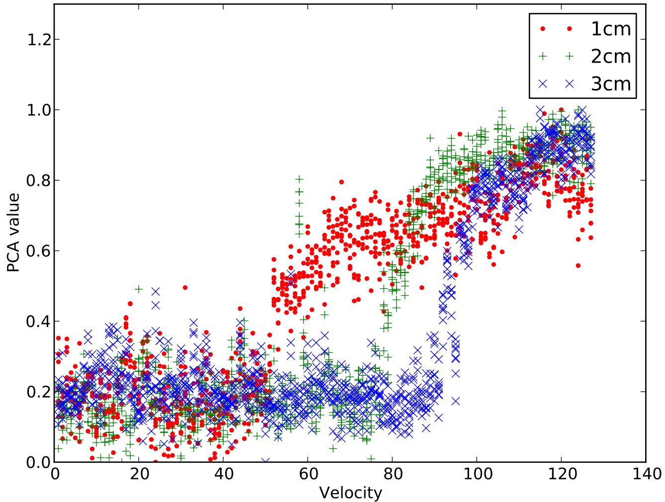
Original PCA Values
